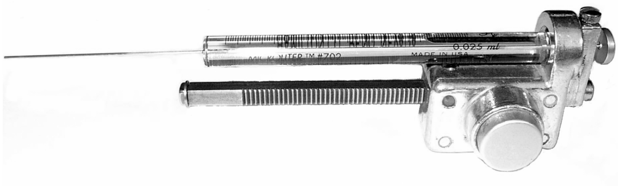
図2 ハミルトン製ディスペンザー
