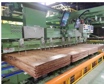
〔合板用乾燥施設〕
