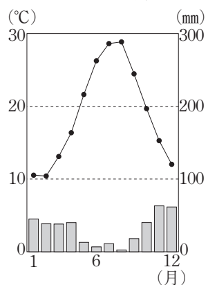
図 1 ある地点の気温と降水量
