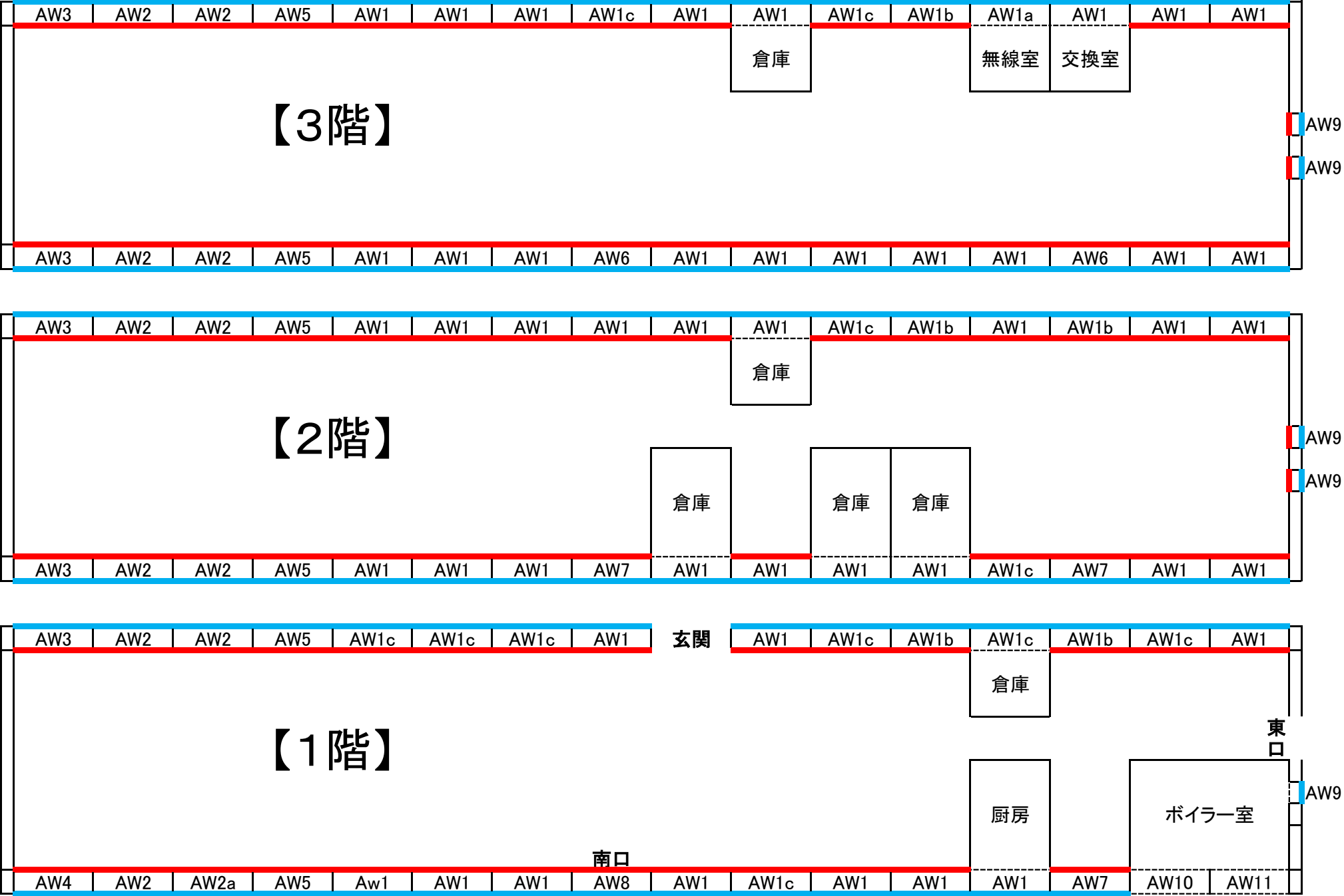
由利地域振興局庁舎清掃窓指定図
