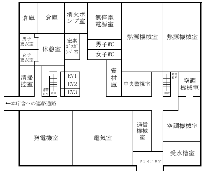
地下2階
