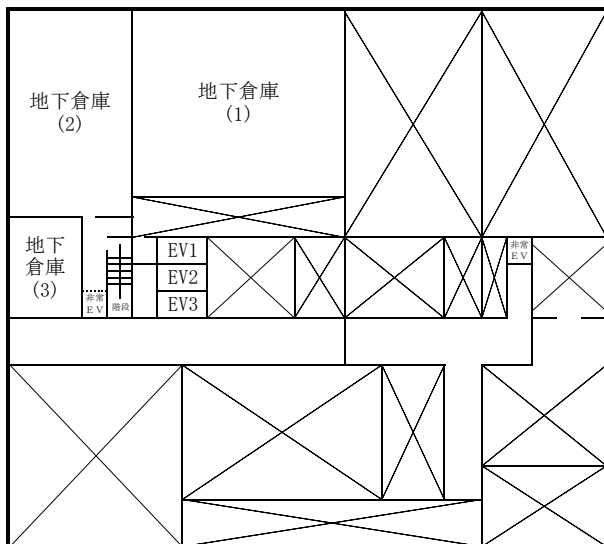
地下1階
