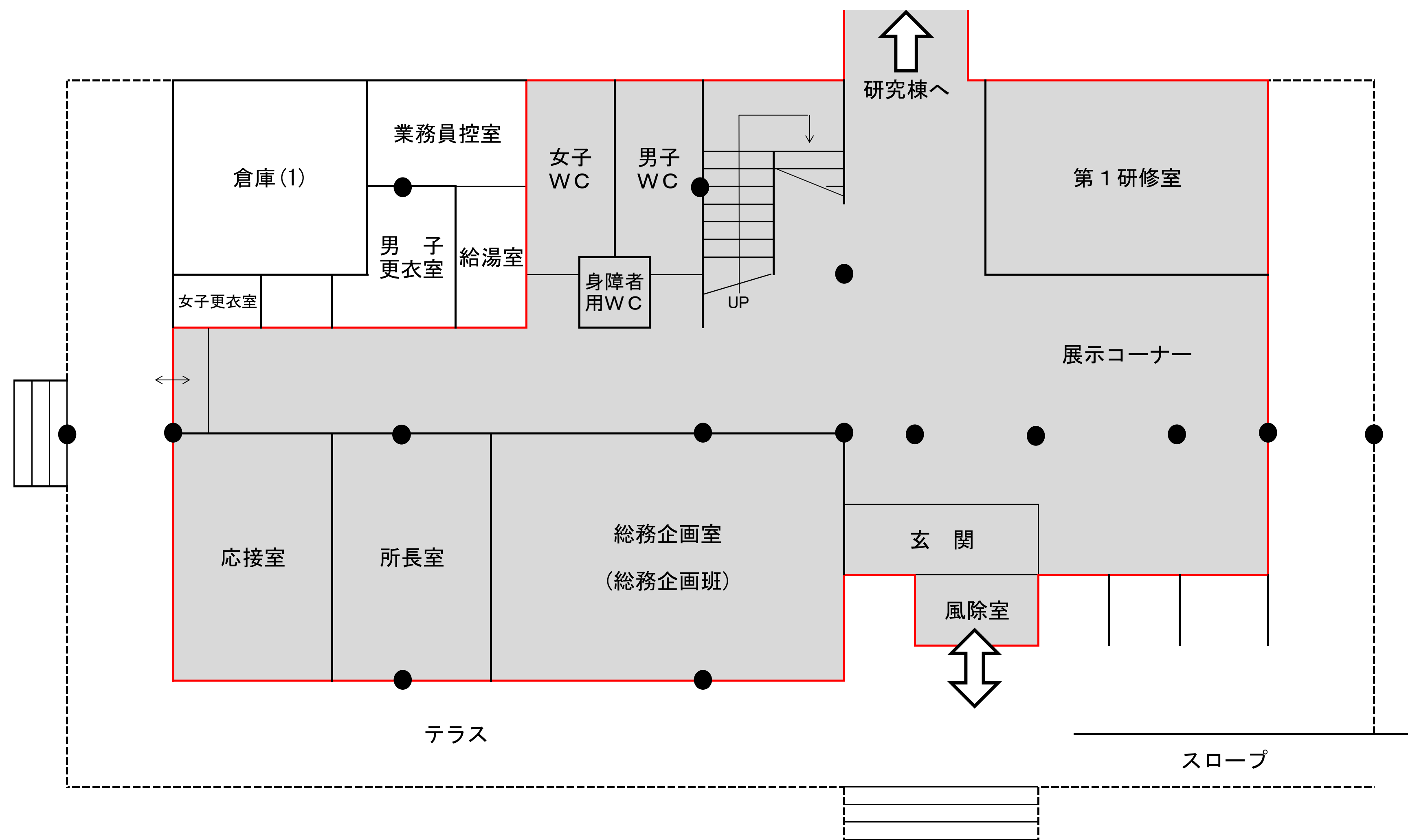
秋田県林業研究研修センター管理棟平面図
