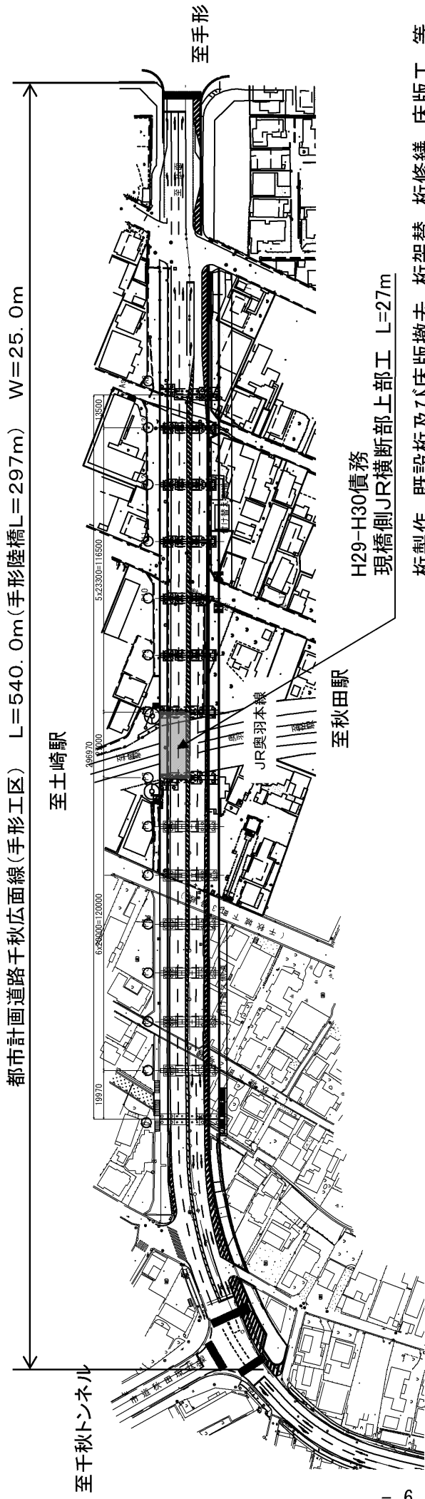
平面図
