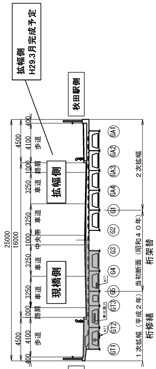
断面図
