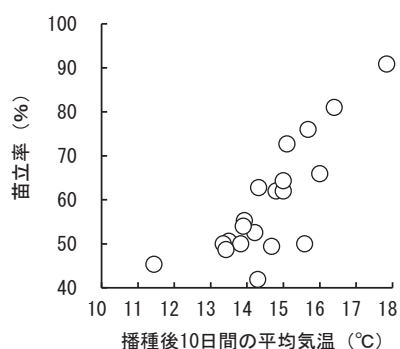
図-3 播種後10日間の平均気温と苗立率の関係 (2002~2021年)
