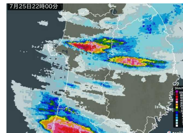
雨量レーダーエコー（7月25日 22時00分）
