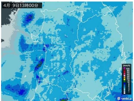
雨量レーダー（4月9日 13:00）
