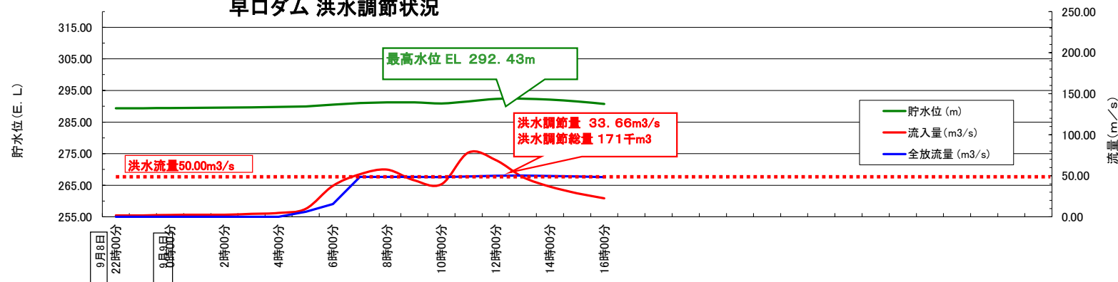
早口ダム 洪水調節状況
