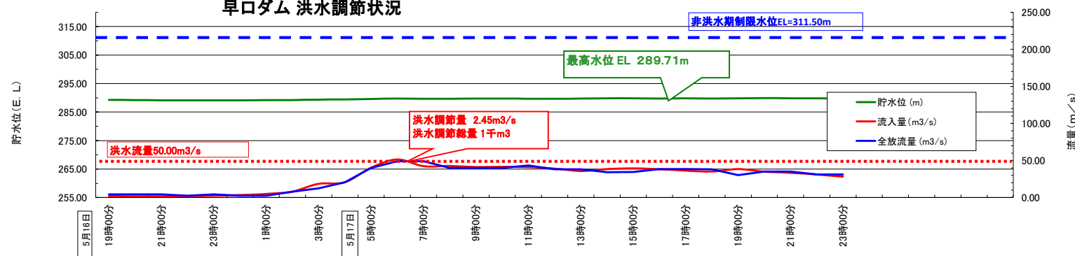
早口ダム 洪水調節状況
