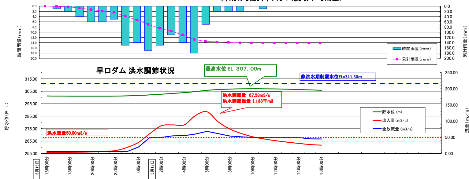
降雨の状況(早口ダム流域平均雨量)
