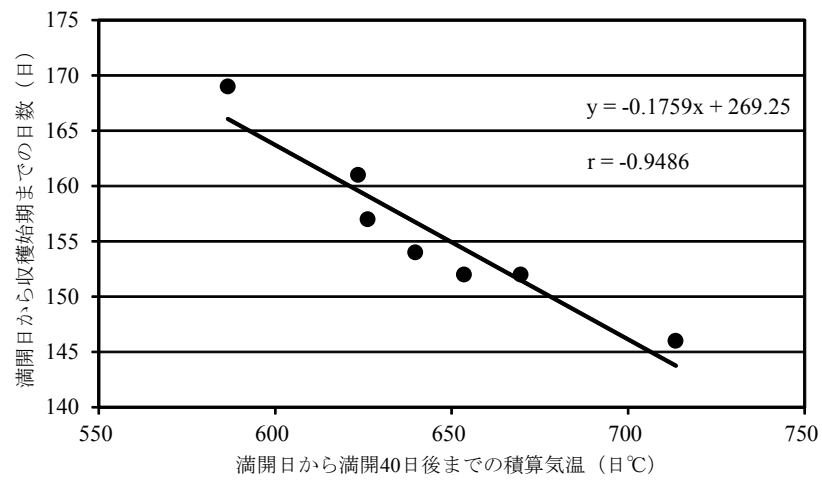
図2 満開日から満開40日後までの積算気温と収穫始期までの日数との関係
