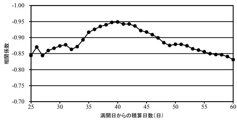
図1 満開日からの積算気温と収穫始期までの日数との相関係数（2008～2014年、天王分場）
