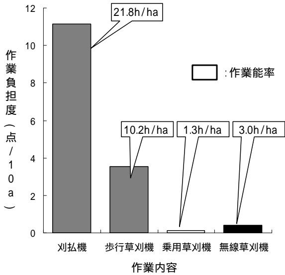
図1 各作業機での草刈作業効率と作業負担度
