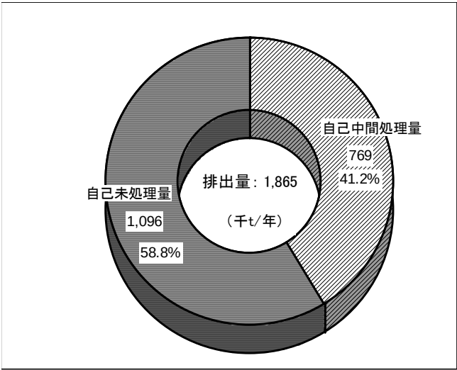
図 2-3-4 中間処理及び自己未処理量の構成比
