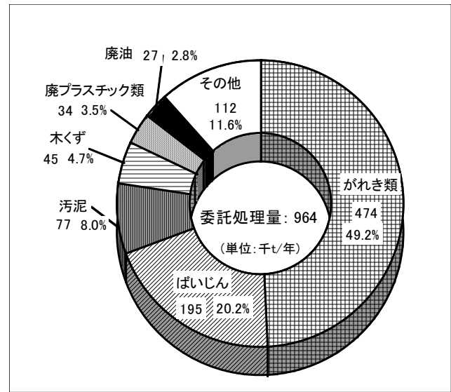
図 2-3-6 種類別委託処理量の構成比
