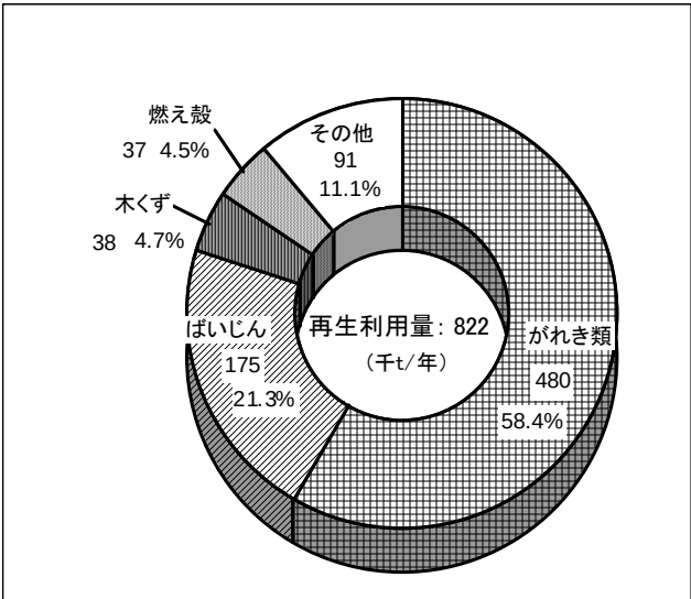
図 2-3-10 種類別の再生利用量の構成比
