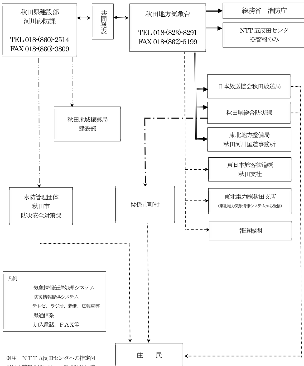
太平川洪水予報伝達系統図
