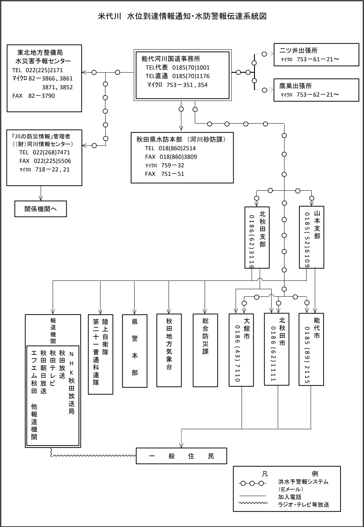
資料5－6 直轄河川水位到達情報通知・水防警報伝達系統図(能代河川国道事務所)
