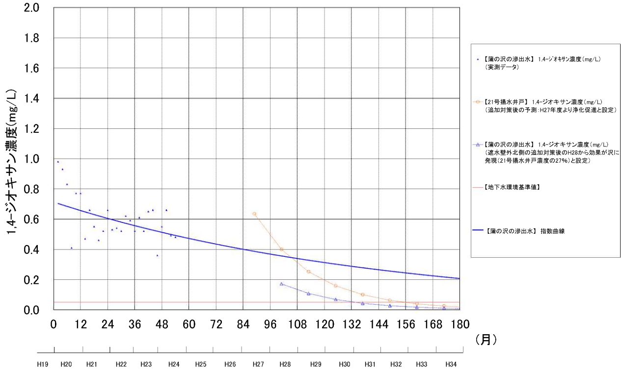
図13 蒲の沢への滲出水 1，4－ジオキサン濃度予測図
