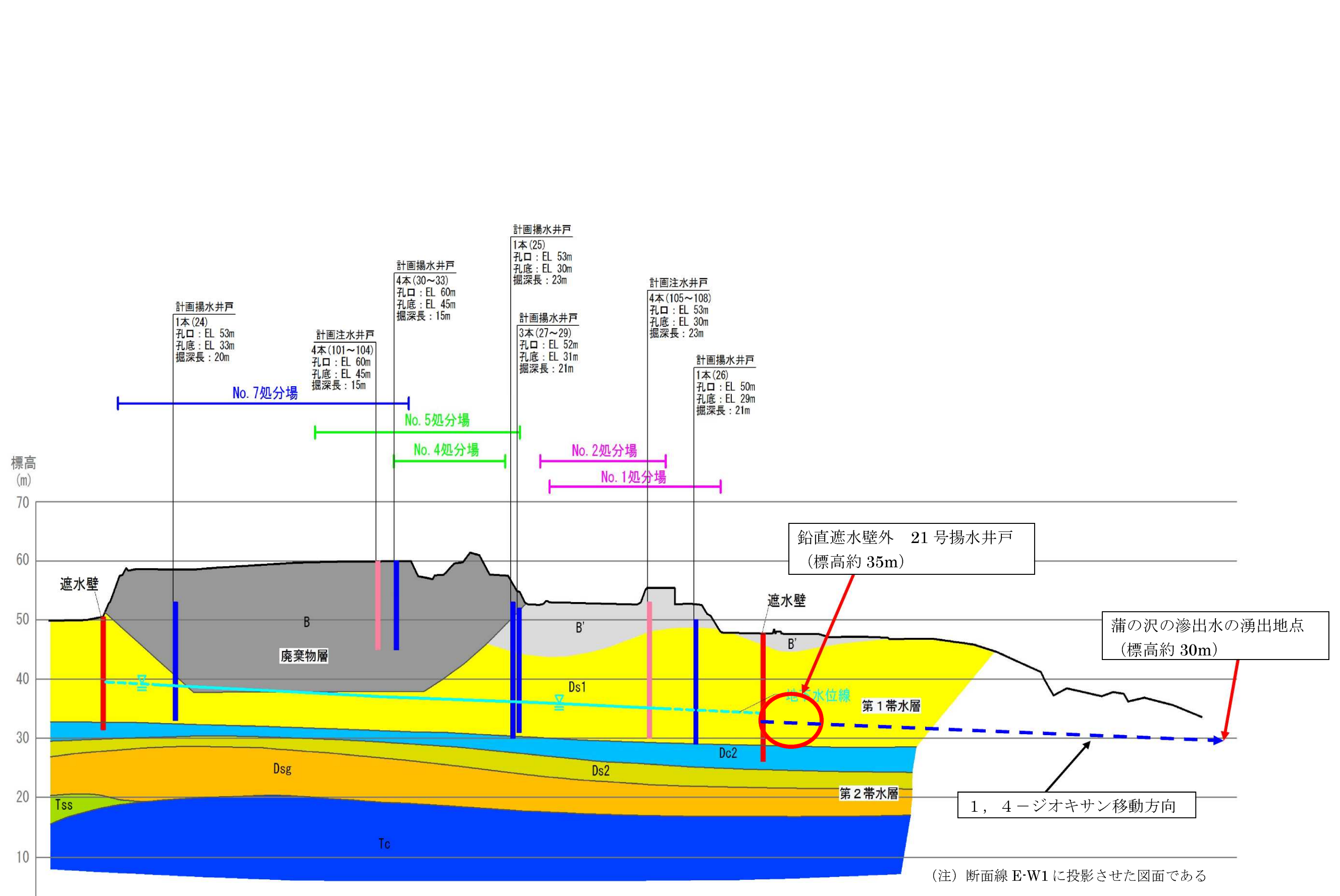
図 1 2 検討位置平面図・断面図
