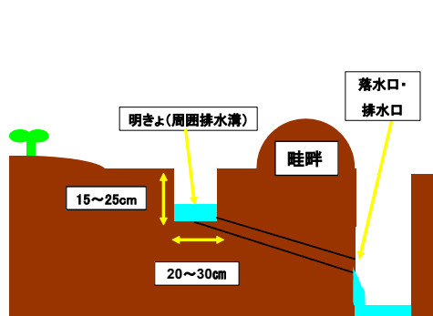
図3 明きよから排水路への排水
