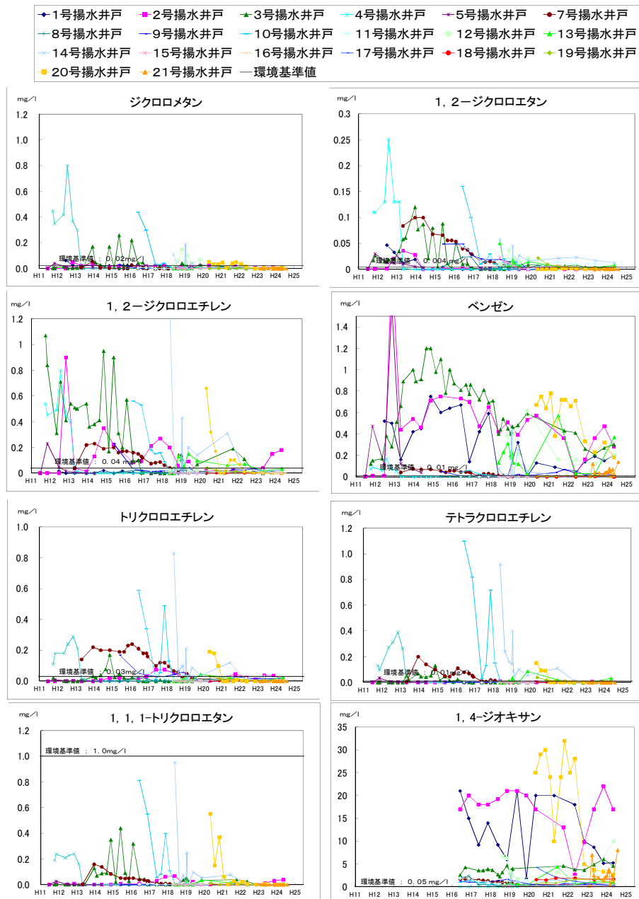
図-5-1 地下水質(揚水井戸)の経年変化
