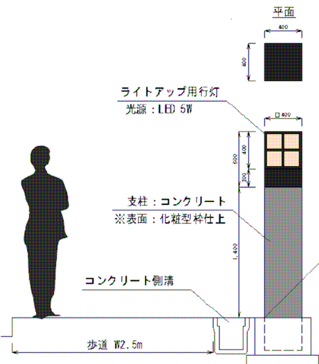
あんどん風照明例
