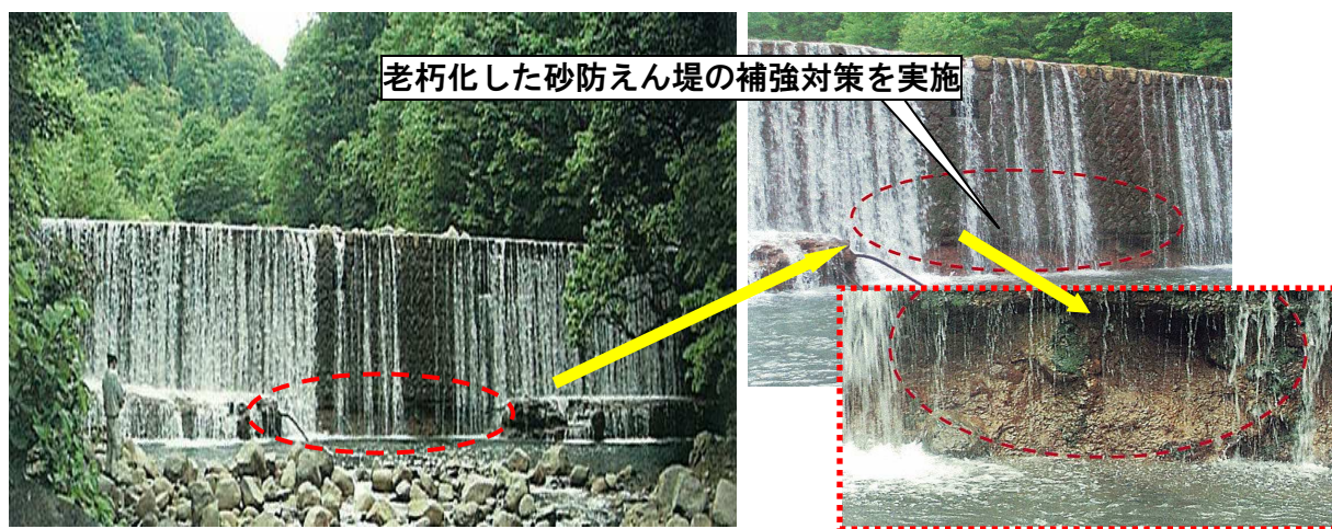
○老朽化対策[総合流域防災事業 熊沢川砂防えん堤（鹿角市）]
