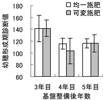
図1 基盤整備後年数と可変施肥が生育及び収量に及ぼす影響(2002~2004年) 注1) 診断値は草丈×莖数×葉緑素計値×10 -4 注2) エラーバーは標準偏差
