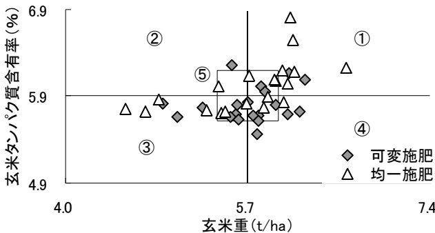
図3 基盤整備後2年目ほ場における玄米重と玄米タンパク質含有率の関係(2005年) 注1) 調査方法は表2と同じ 注2) 図中の目盛り線は平均値, 中央部罫線は平均値±5%の範囲
