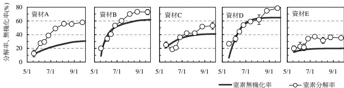
図2 水稻作付期間中における各有機質資材の窒素分解率と窒素無機化率の推移
