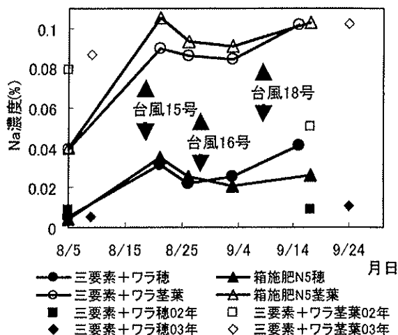
第11図 潮風害前後の部位別Na濃度の推移 (秋田農試大潟試験地、2004)
