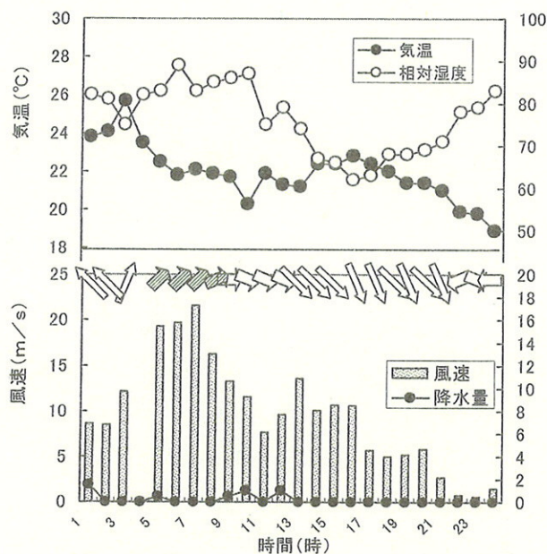
第6図 台風15号通過に伴う気象要素の経過
