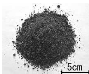
溶融スラグ
