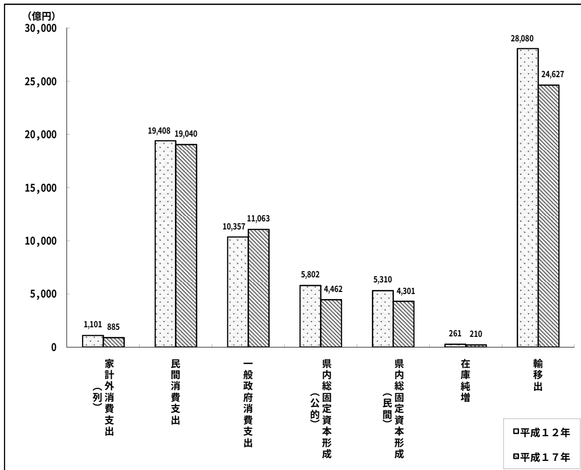
図 1 - 1 4 生産誘発額
