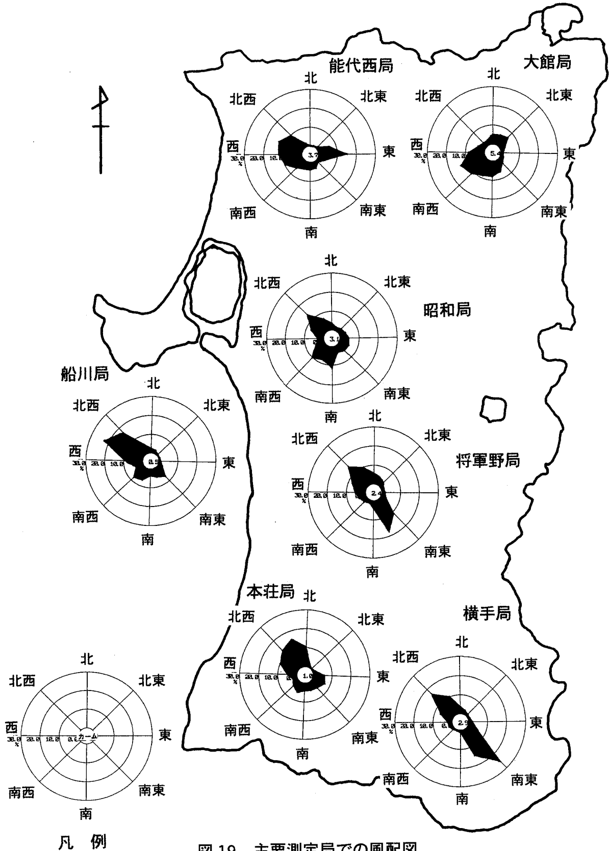
図 19 主要測定局での風配図
