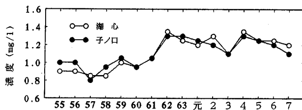
図2 十和田湖のCODの経年変化(75%値)
