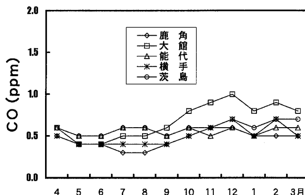
図 18 一酸化炭素月平均値の変化
