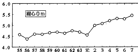
図4 田沢湖のpHの経年変化(平均値)
