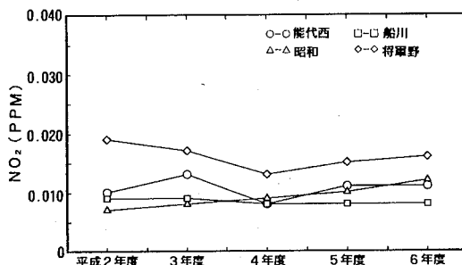
図6 主要測定局での二酸化窒素日平均値の年間98%の推移
