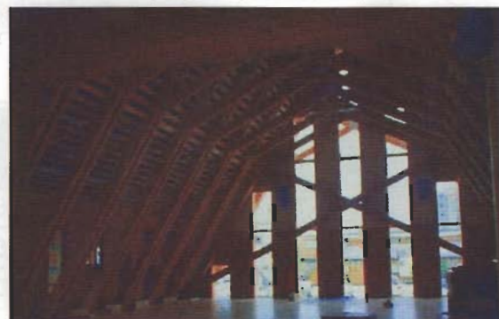
秋田杉の大断面集成材を使用したトラス構造
