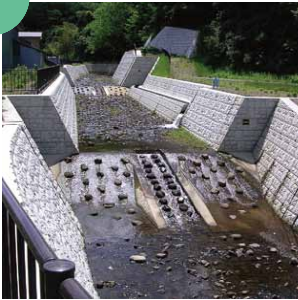
自然石を活用し魚道など整備して、生態系と環境に配慮した砂防えん堤。 (にかほ市・寒沢川)
