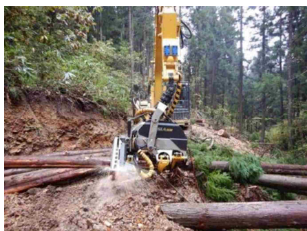
ハーベスタ作業（伐木・造材）
