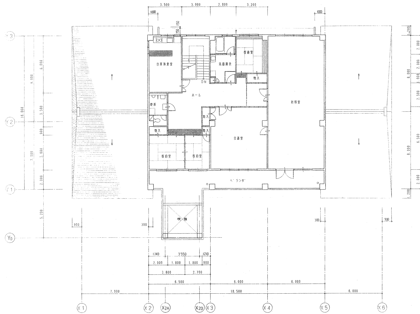
2階 平面図 1/100
