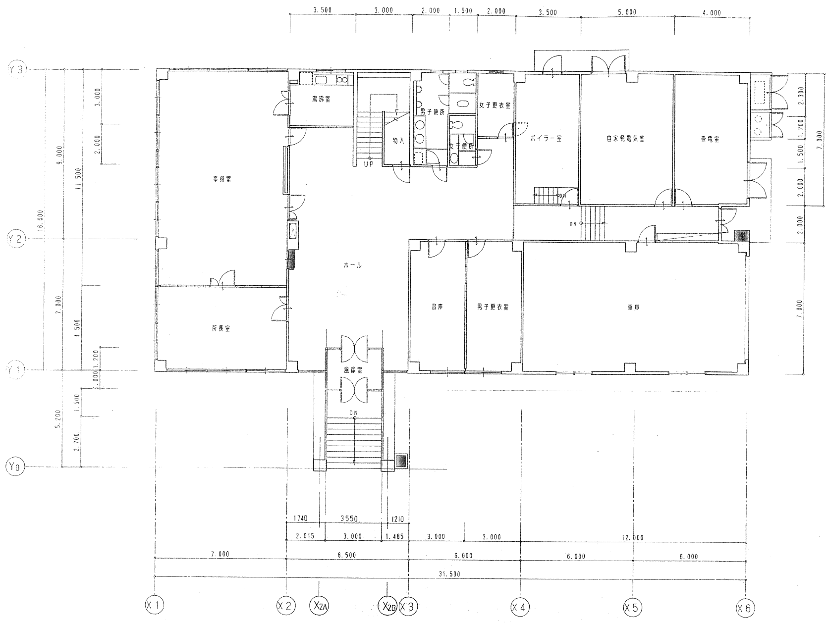
1階 平面図 1/100
