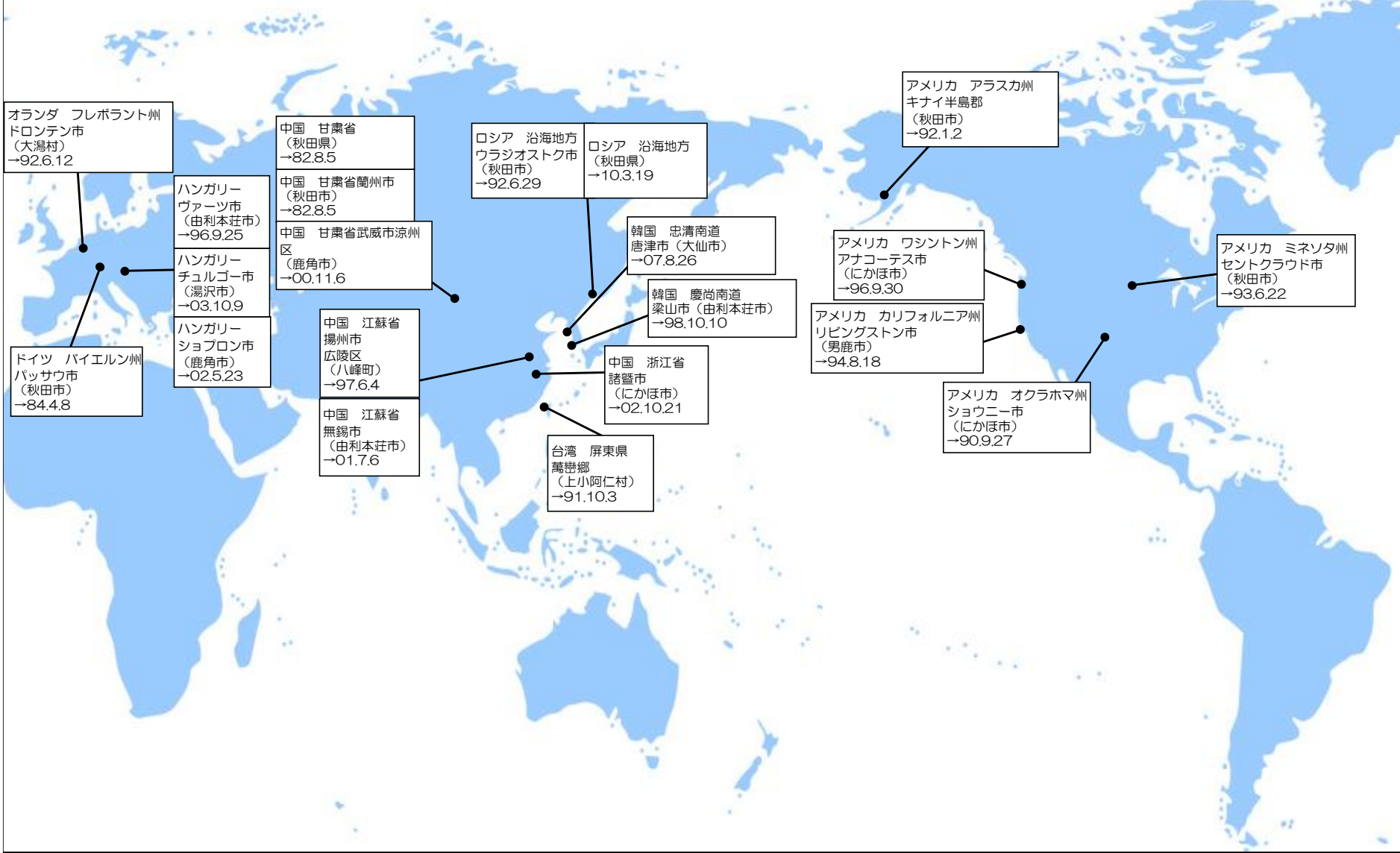
図2 海外との友好・姉妹都市提携の状況（世界地図）（平成30年3月末現在）
