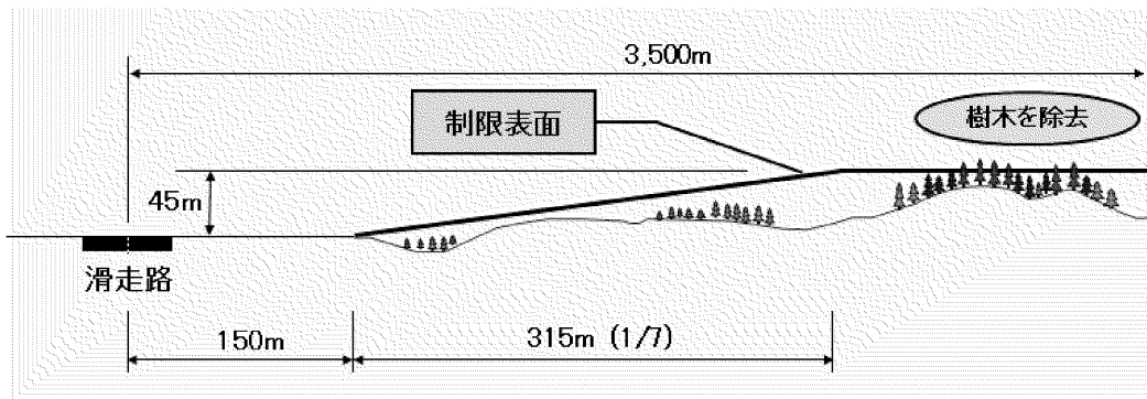
制限表面イメージ図（秋田空港）
