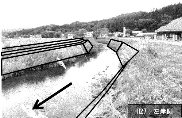
県単河川改良事業 楡木内川（仙北市） 築堤・護岸工
