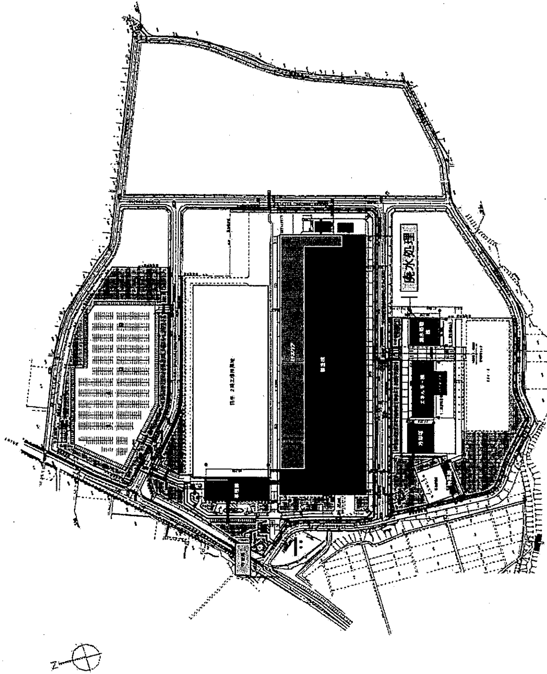
TDK秋田桐本荘工場 西サイト 配置図
