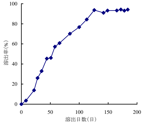
図2 肥効調節型肥料 70日タイプの溶出パターン
