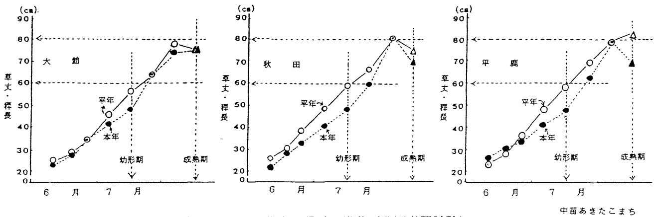
第Ⅲ-6図 草丈・稈長の推移(豊凶考照試験)
