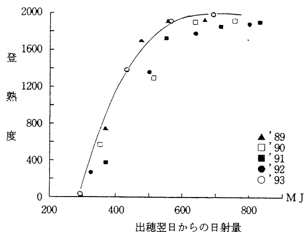
第VI-41図 出穂翌日からの日射量と登熟度
