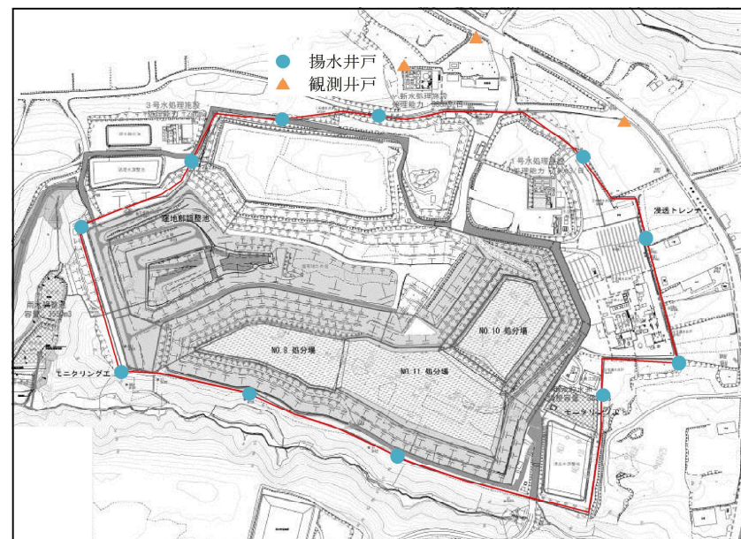
第2帯水層を対象とした井戸の位置図
