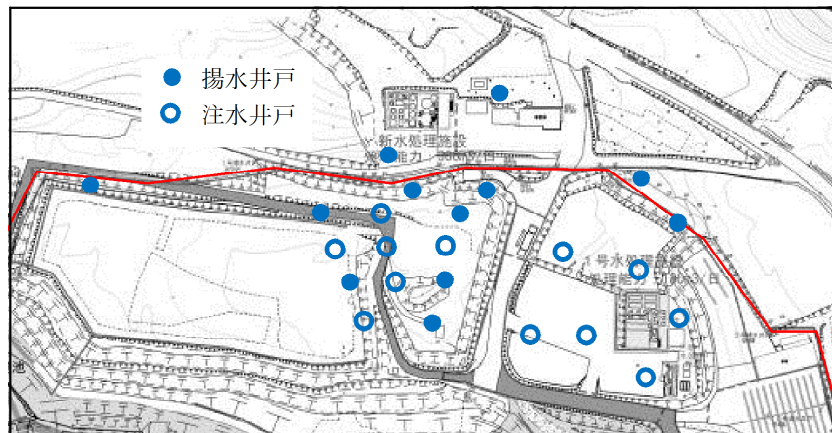
第1帯水層を対象とした井戸の位置図
