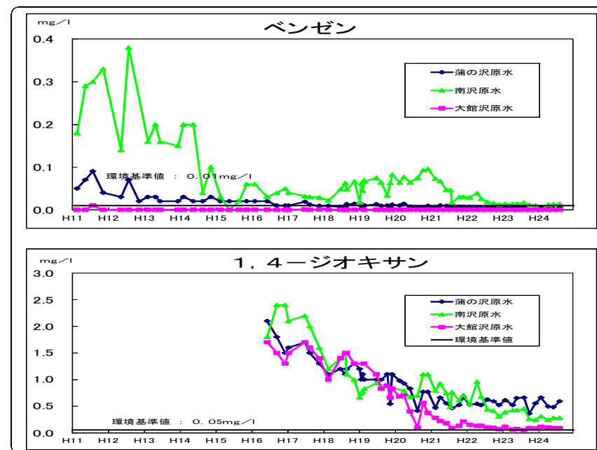
蒲の沢、南沢及び大館沢滲出水の主なVOCの経年変化
