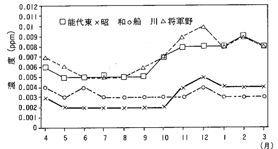
図7 平成3年度主要測定局における二酸化窒素の経月変化 (月平均値)
