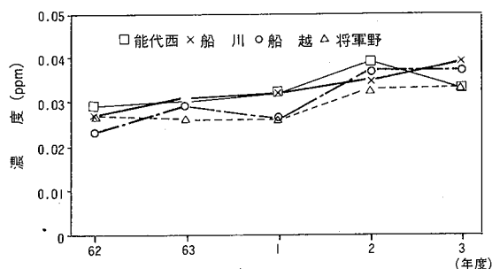
図 8 オキシダントの経年変化 (昼間の 1 時間値の年平均値)
