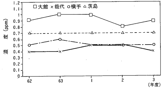
図15.1 主要測定局における一酸化窒素の経年変化 (年平均値)
