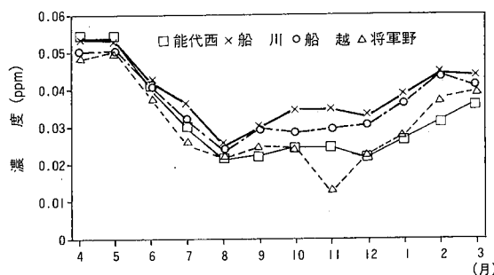
図 9 平成 3 年度オキシダントの経月変化 (昼間の 1 時間値の月平均値)
