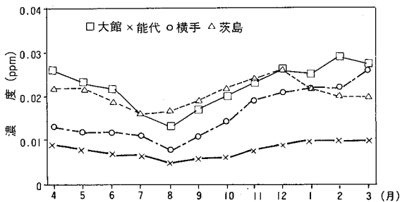
図14.2 平成3年度主要測定局における二酸化窒素の経月変化 (月平均値)
