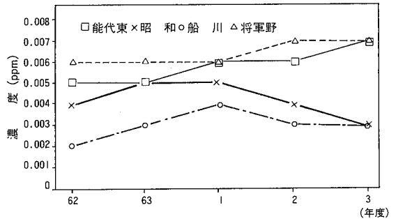
図5 主要測定局における二酸化窒素の経年変化 (年平均値)
