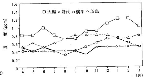
図15.2 平成3年度主要測定局における一酸化窒素の経月変化 (月平均値)
