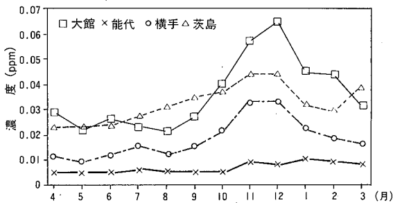
図14.1 平成3年度主要測定局における一酸化窒素の経月変化 (月平均値)
