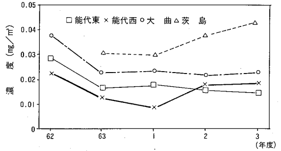
図11 主要測定局における浮遊粒子状物質の経年変化 (年平均値)
