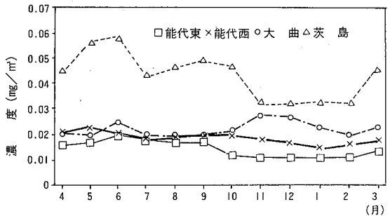
図12 平成3年度主要測定局における浮遊粒子状物質の経月変化 (月平均値)
