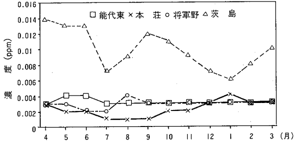
図4 平成3年度主要測定局における二酸化硫黄の経月変化 (月平均値)
