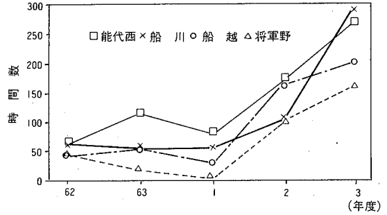
図10 オキシダント1時間値が0.06ppmを超えた時間数
