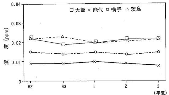
図13.2 主要測定局における二酸化窒素の経年変化 (年平均値)
