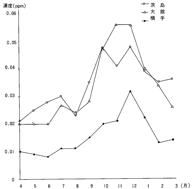
図-15-1 昭和62年度主要測定局の一酸化窒素経月変化 (月平均値)
