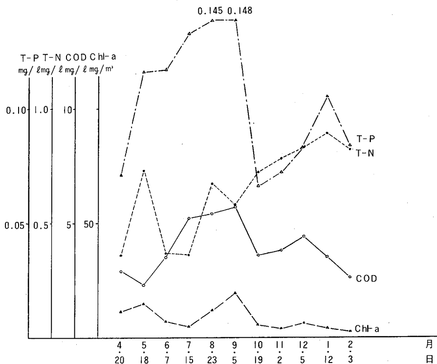
図一六 防潮水門における経月変化（表層）
