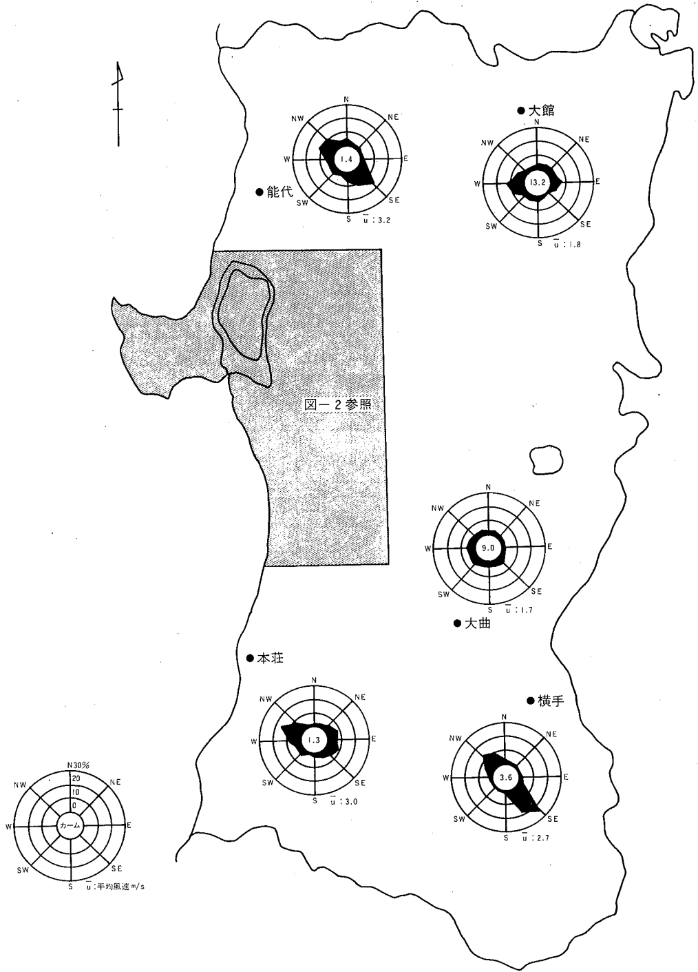
図-1 風配図
