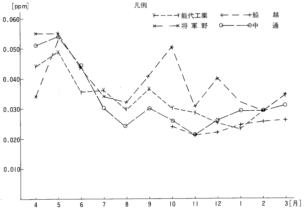
図-12 昭和58年度オキシダント濃度(昼間の日最高1時間値)の月別変化
