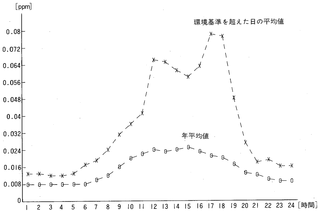
図一3 環境基準を超えた日の時刻別変化
