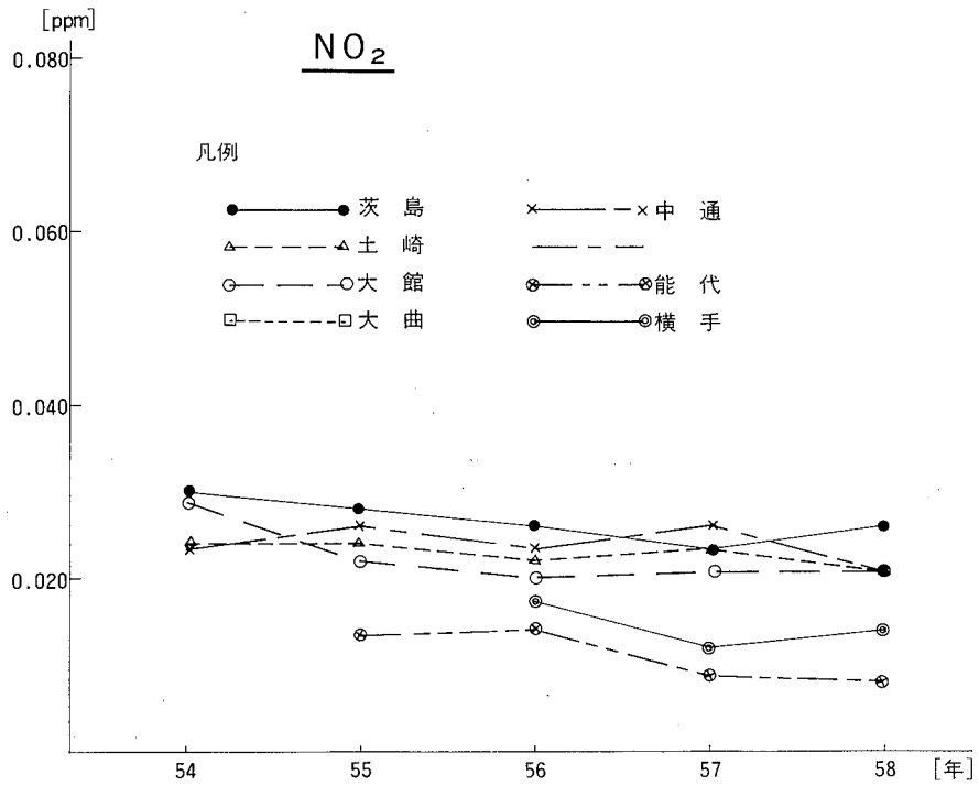
図一八 窒素酸化物濃度の経年変化
