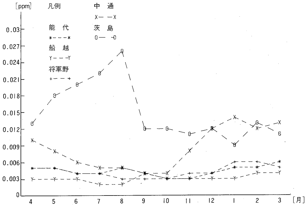
図一六 昭和58年度主要測定局の二酸化硫黄濃度月別変化
