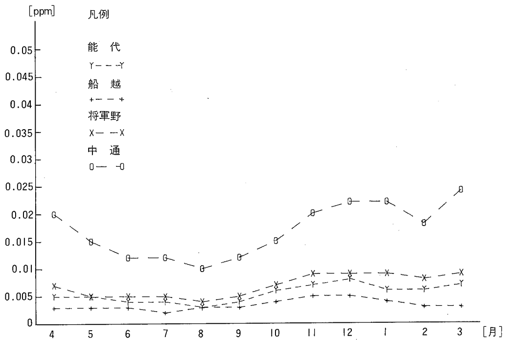
図一八 昭和58年度主要測定局の二酸化窒素濃度変化
