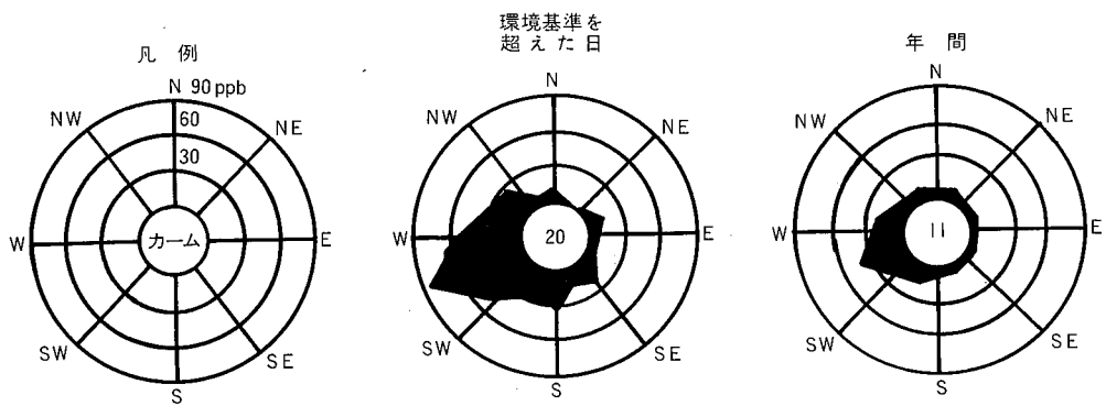
図一4 環境基準を超えた日の風向別濃度変化
