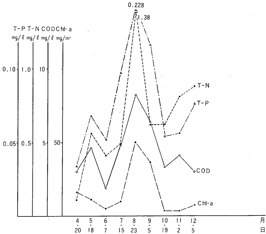
図一五 調整池中央における経月変化（表層）
