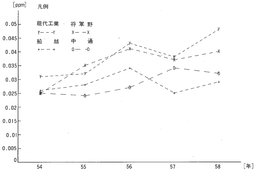
図-10 オキシダント濃度の経年変化（昼間の日最高1時間値の年平均値）
