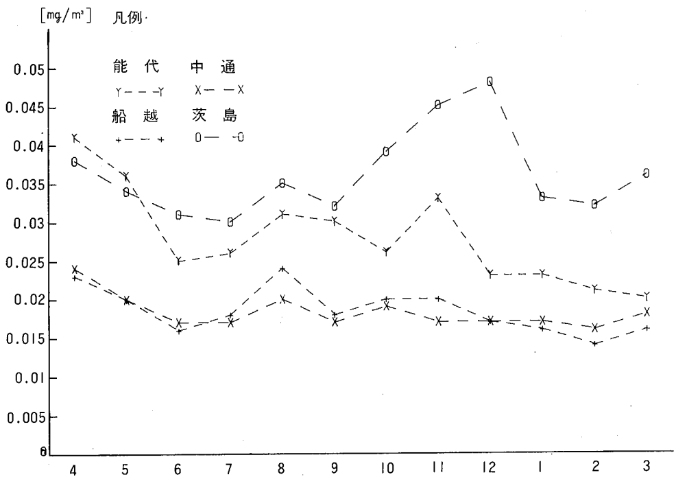
図一17 昭和58年度主要測定局の浮遊粉じん濃度月別変化
