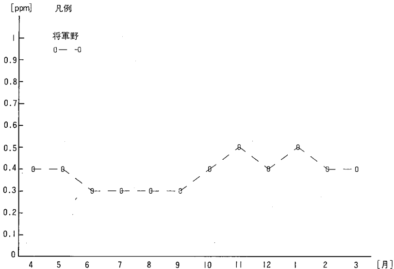
図一9 昭和58年度一酸化炭素濃度の月別変化
