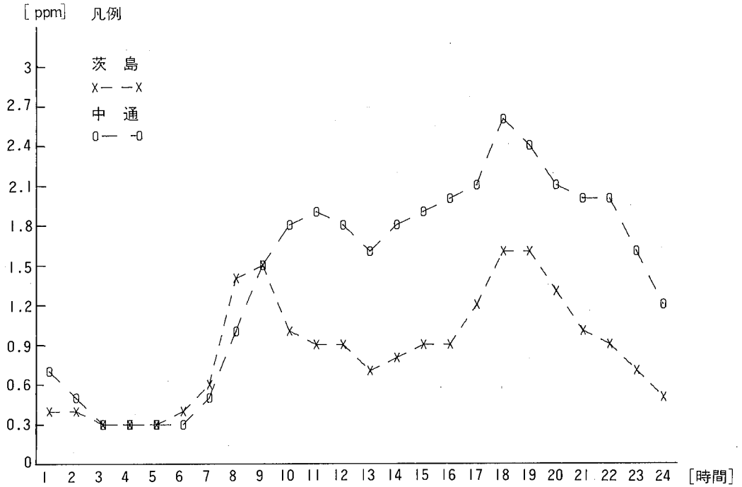
図-21 昭和58年度一酸化炭素濃度の時刻別変化
