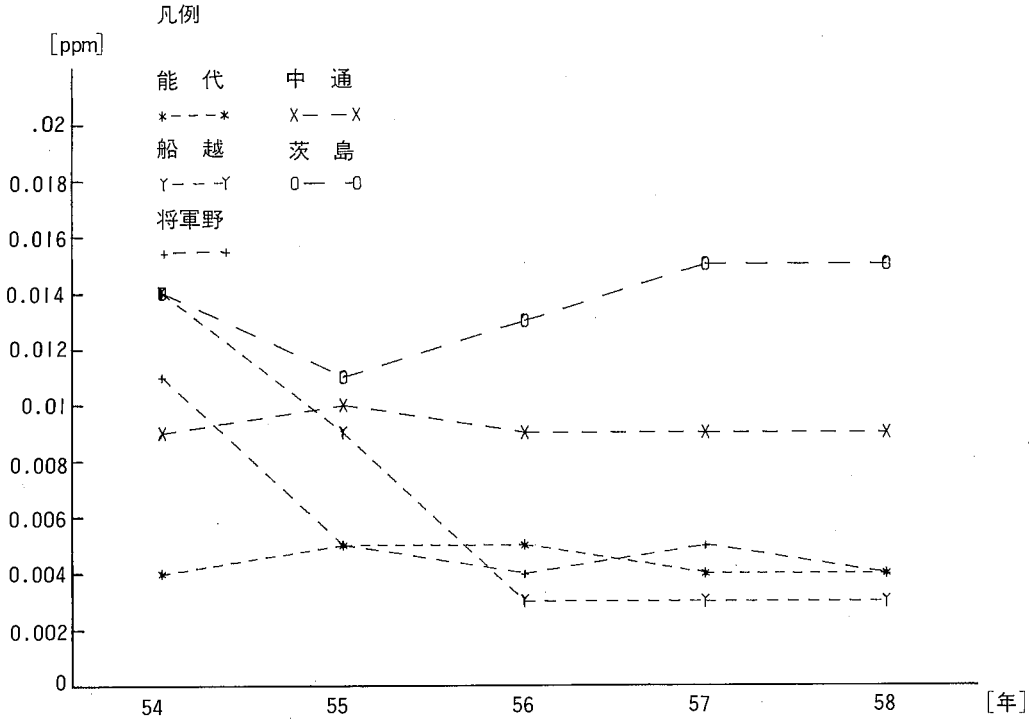
図一五 主要測定局の過去5年間の二酸化硫黄濃度変化
