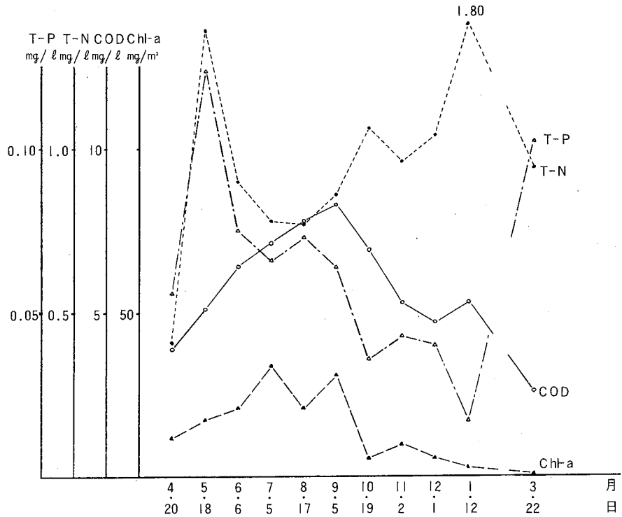
図一 3 浜口排水機場における経月変化
