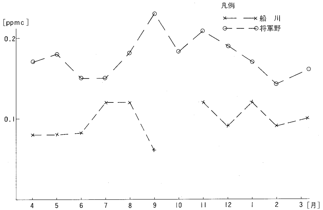
図-14 昭和58年度非メタン炭化水素濃度の月別変化
