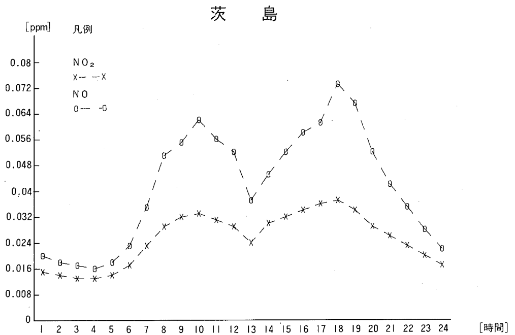
図一19 昭和58年度窒素酸化物濃度の時刻別変化
