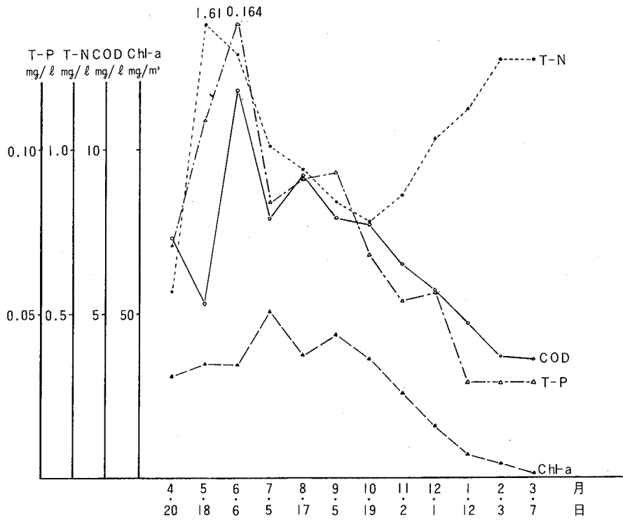
図一 2 野石橋における経月変化
