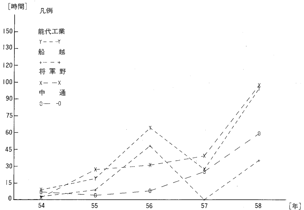
図-11 オキシダント濃度1時間0.06ppmを超えた時間数の経年変化
