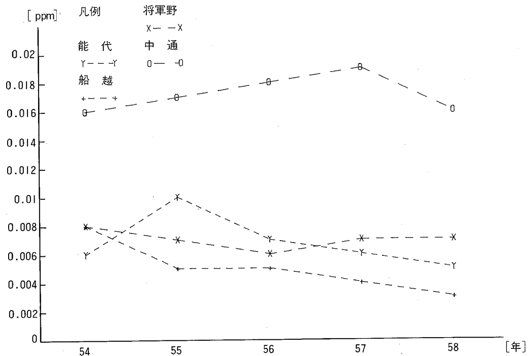
図一七 主要測定局の過去5年間の二酸化窒素濃度変化
