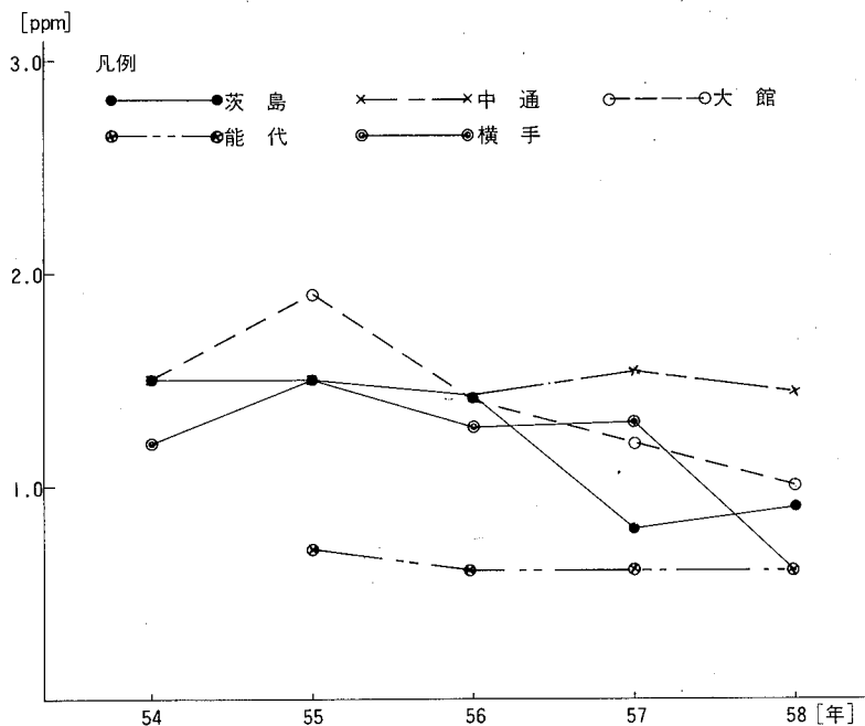
図-20 一酸化炭素濃度の経年変化
