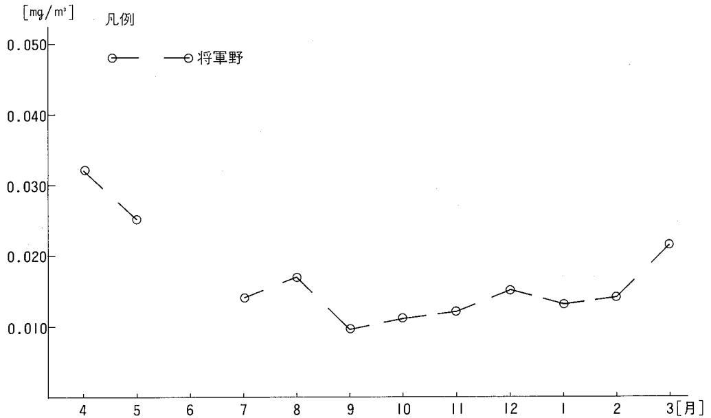
図-15 昭和58年度浮遊粒子状物質濃度の月別変化 (將軍野局)
