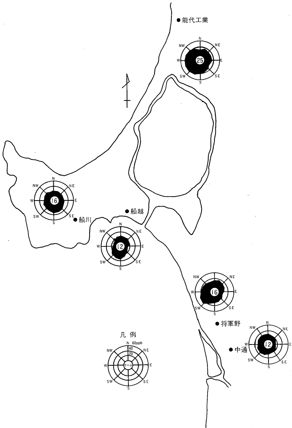
図-13 昭和58年度風向別オキシダント濃度
