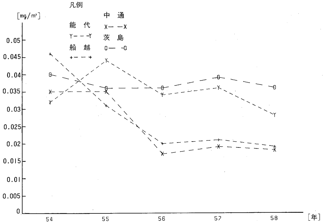
図一16 主要測定局の浮遊粉じん濃度経年変化
