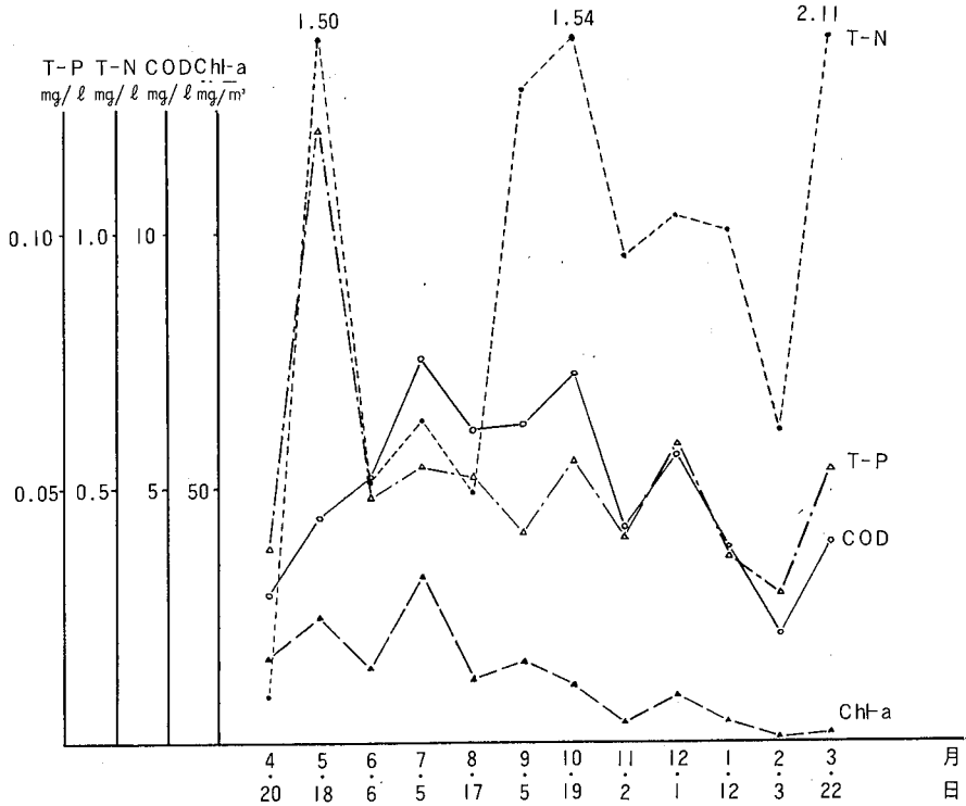
図一四 大瀧橋における経月変化（表層）
