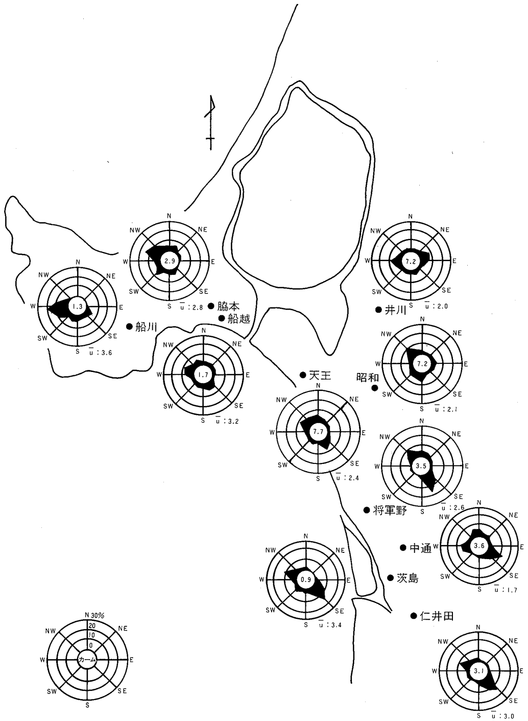
図-2 風配図
