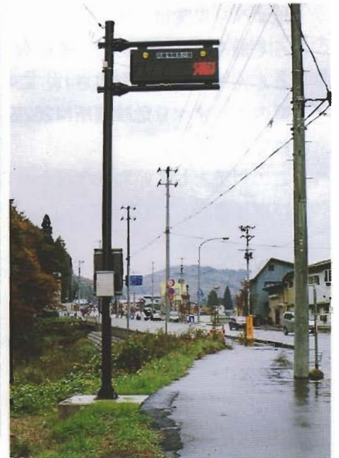
《土砂災害危険箇所の集中する地域に設置し住民に雨量情報を知らせる雨量表示板 湯沢市》
